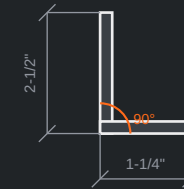
Nez de marche (coupe)
